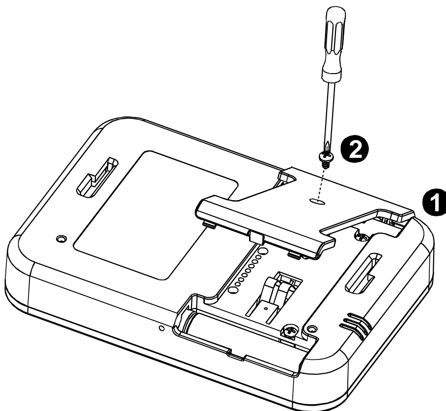
Figuur 2 – Batterij klep plaatsen (optie a)
