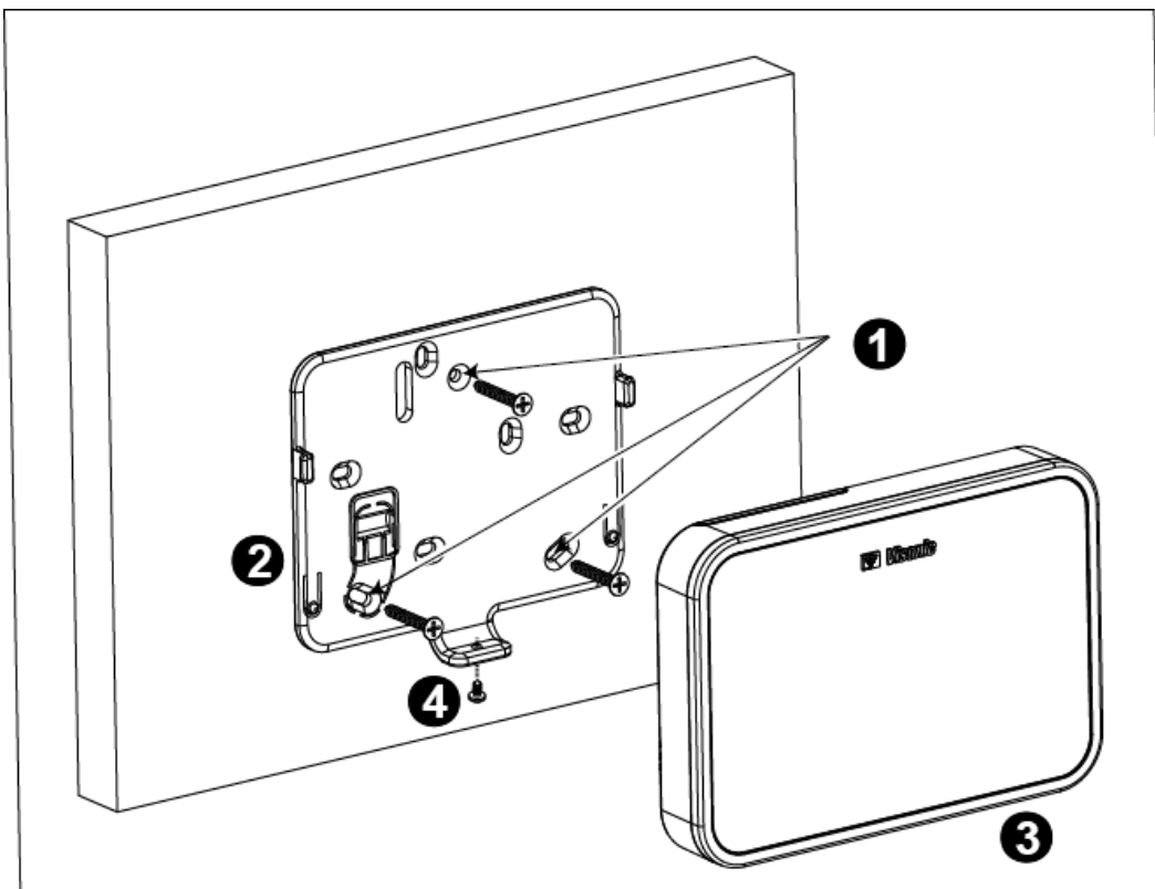
Figuur 4a – Wandmontage
