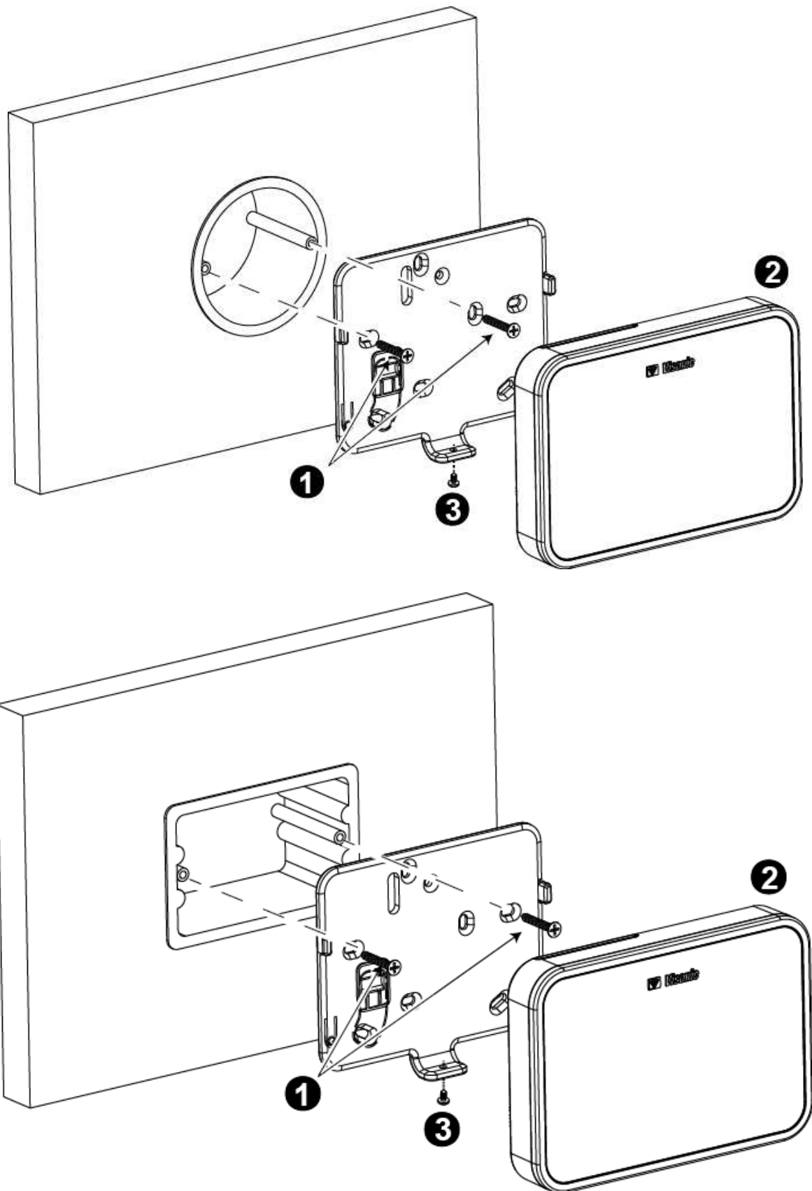
Figuur 4b – Wandmontage met externe voeding
