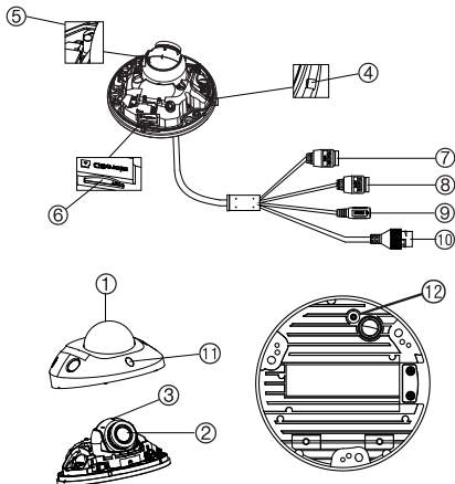
Afbeelding 7: IP wedge camera met vaste lens
