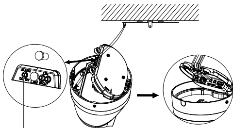
Zwart rubberen inzetstuk
